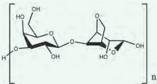
Structura chimică a agarului
